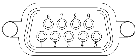
8-1 腳位配置
