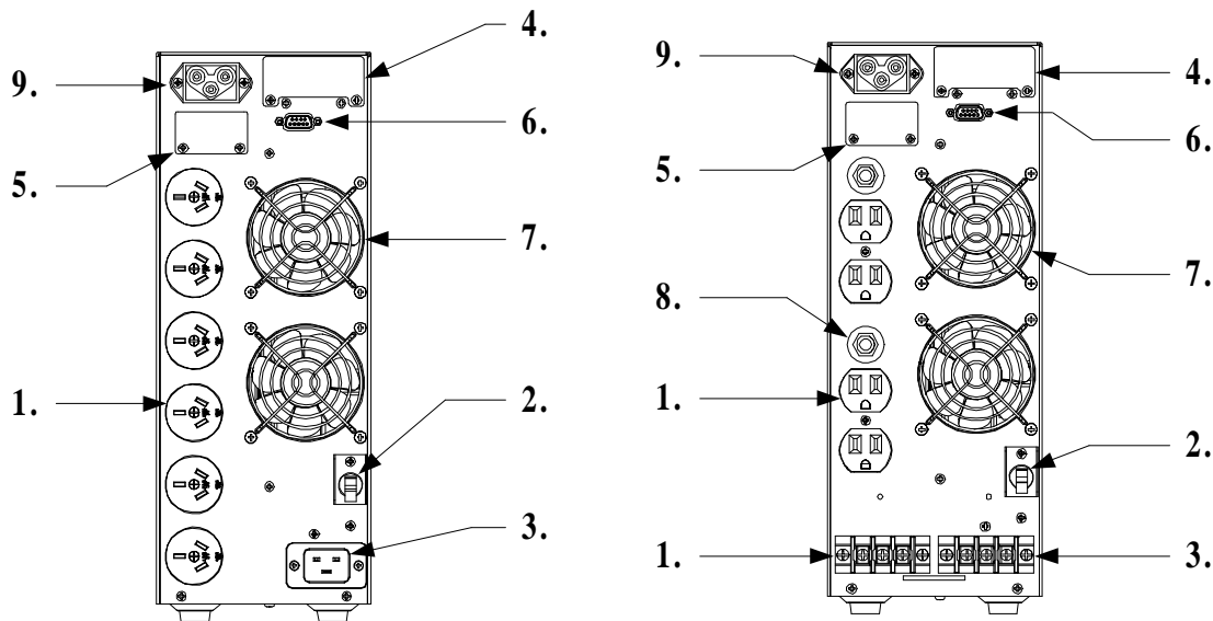
2-4 2KVA , 3KVA 機種的後面板
