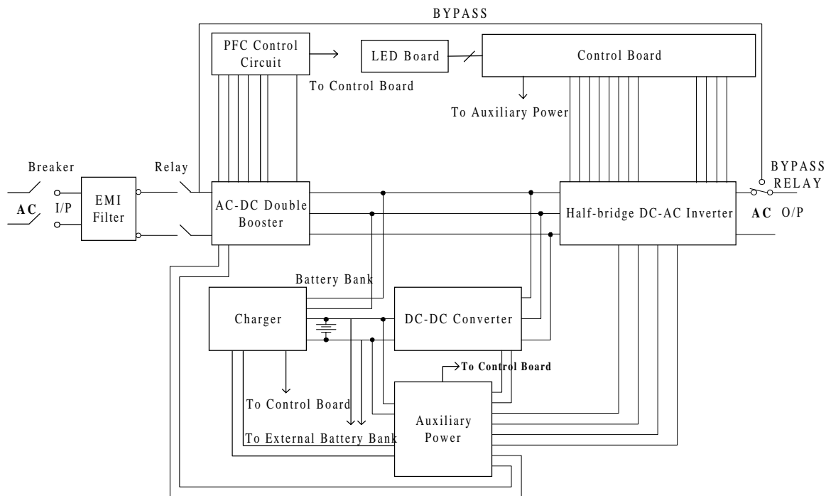
2.1 UPS 系統方塊圖
