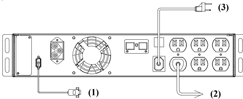
图 3-4 UPS 連接
