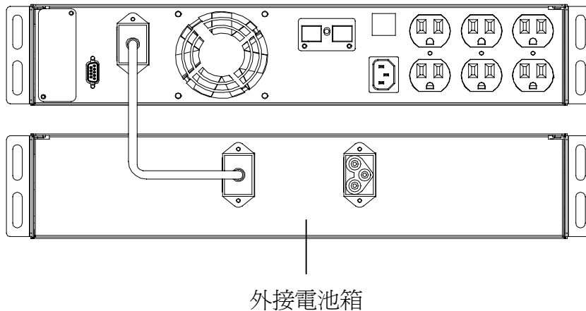
图 3-3 UPS 外接電池箱
