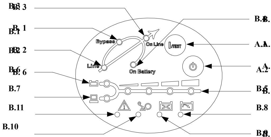
图 2-2 操作面板
