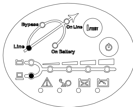
图 3-1 待機模式
