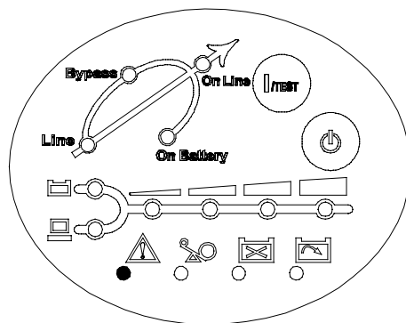
4-8 輸出短路
